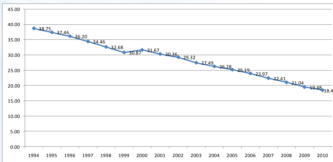
Gráfica 7: Comportamiento del analfabetismo del periodo 1994-2010
